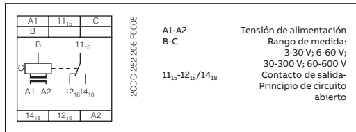
Esquema de conexión CM-ESS.1
