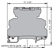
Módulo de abrazadera de resorte
