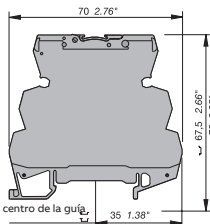
Módulo de abrazadera de tornillo
