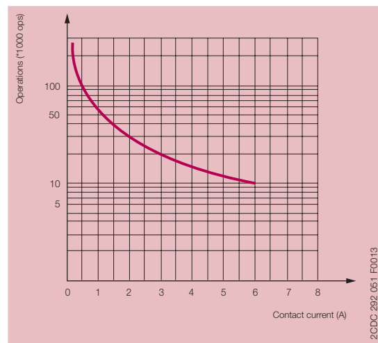
Curva desgaste
