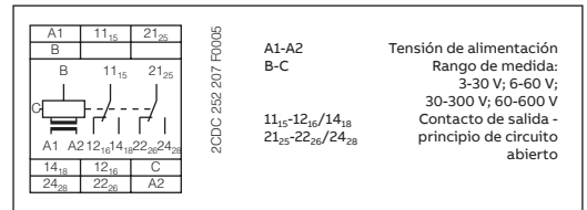
Esquema de conexión CM-ESS.2
