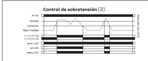
Diagrama de funcionamiento CM-ESS.1
