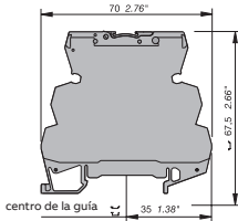
Módulo de abrazadera de tornillo
