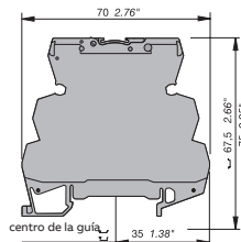
Módulo de abrazadera de tornillo
