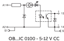
OB...IC 0100 - 5-12 V CC
