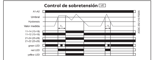
Diagrama de funcionamiento CM-ESS.2
