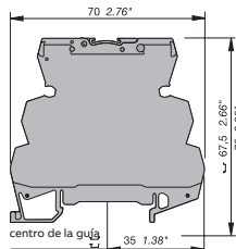
Módulo de abrazadera de tornillo
