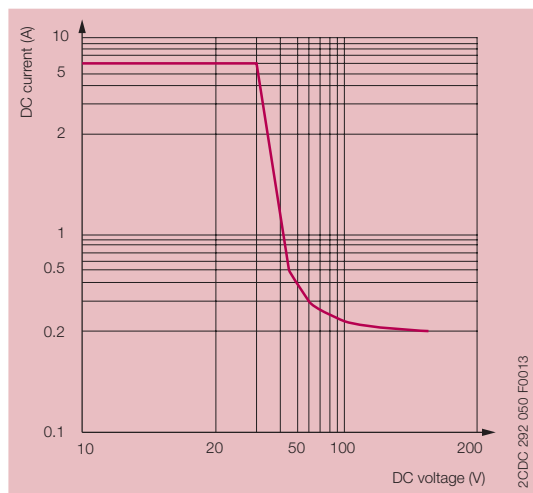
Curva límite máximo de carga
