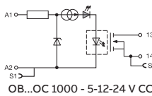
OB...OC 1000 - 5-12-24 V CC
