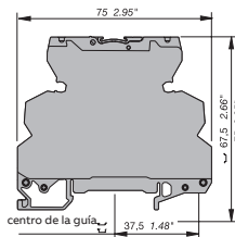
Módulo de abrazadera de resorte
