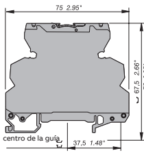
Módulo de abrazadera de resorte
