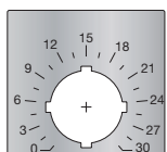
Etiqueta de marcado con escala 0-30 48,5 x 44,5 mm
