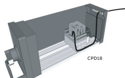
Módulo de comunicación montado sobre armario, montaje remoto.
